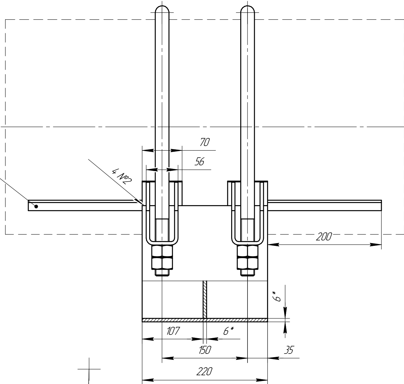
Дет. поз. 6 (1:1)
