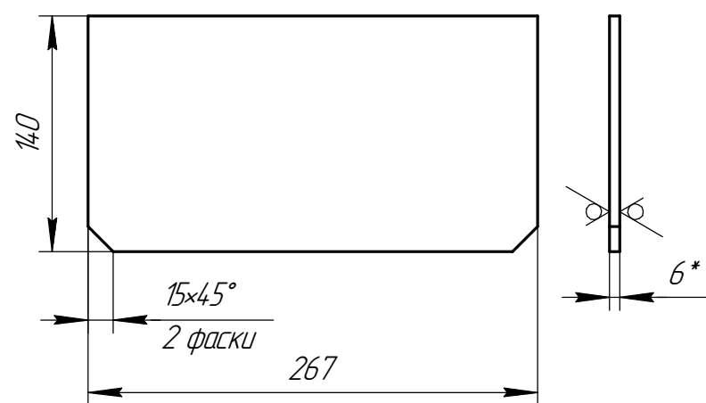
Дет. поз. 2
