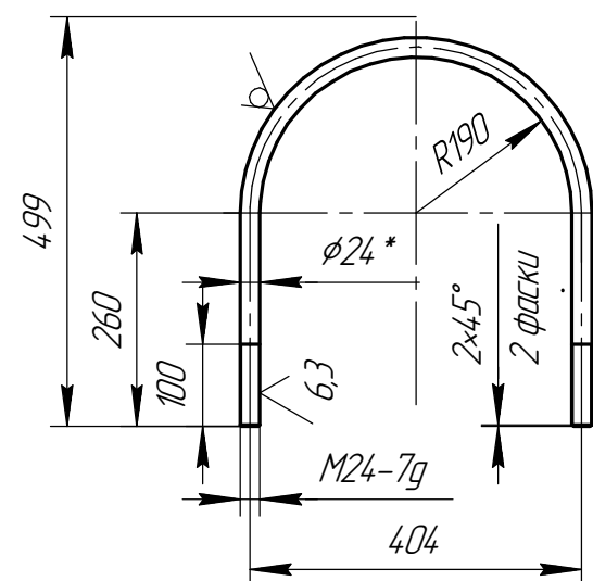
Дет. поз. 5
