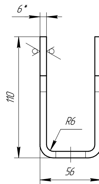
Дет. поз. 3 (1:2)
